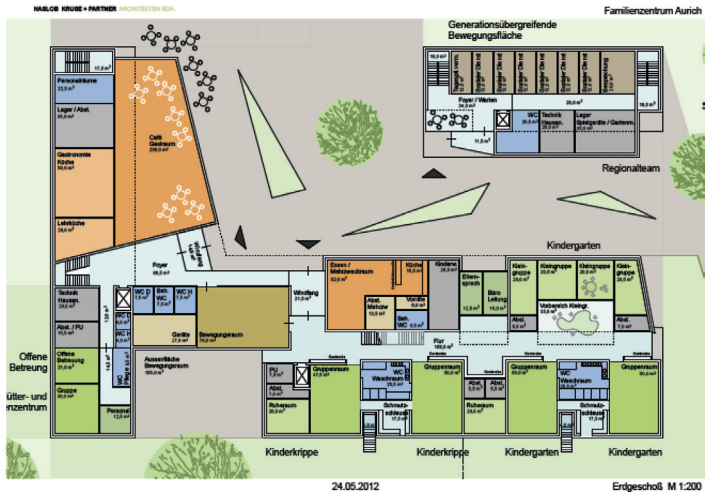
Abbildung: Erdgeschoss Familienzentrum/Mehrgenerationenhaus
