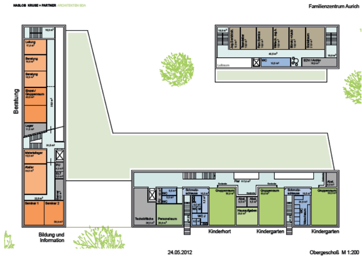
Abbildung: Obergeschoss des Familienzentrums/Mehrgenerationenhauses
